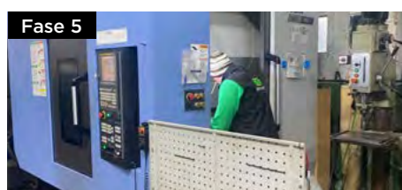
Fase 5 LAVORAZIONE DELL'ANCORA I fori di ancoraggio e di svasatura vengono eseguiti sui CNC.
