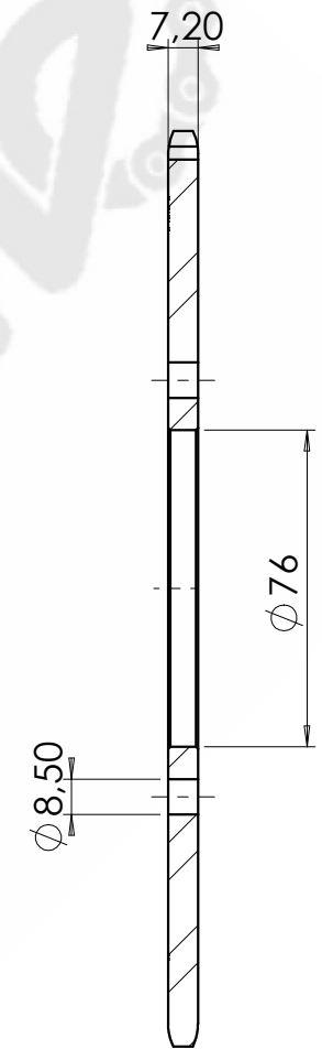
SEZIONE A-A
