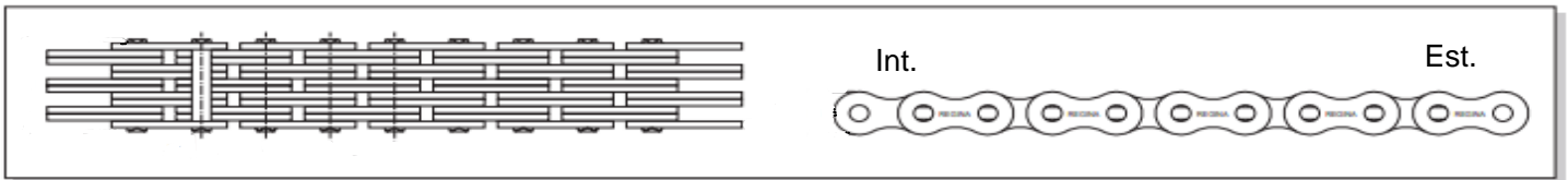
Catena lifter terminali interno - interno
